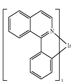
Ir(piq) 3
