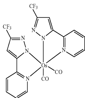
Os(fppz) 2 (CO) 2
