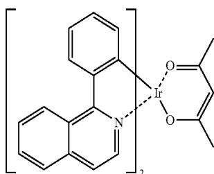
Btp 2 Ir(acac)
