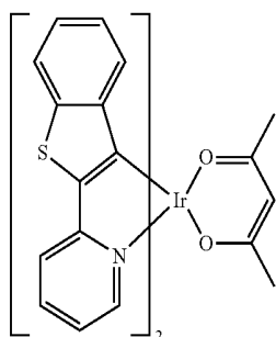
Btp 2 Ir(acac)
